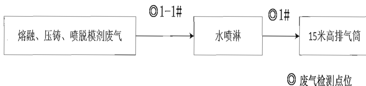
图 3-2 废气处理工艺流程图
