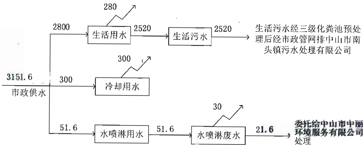
图 2-1 项目实际水平衡图 (单位: t/a)
